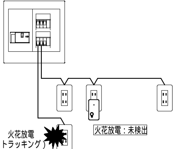
〈他の分岐回路で火花放電が発生した場合〉
