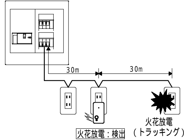
〈同電路上で火花放電が発生した場合〉
